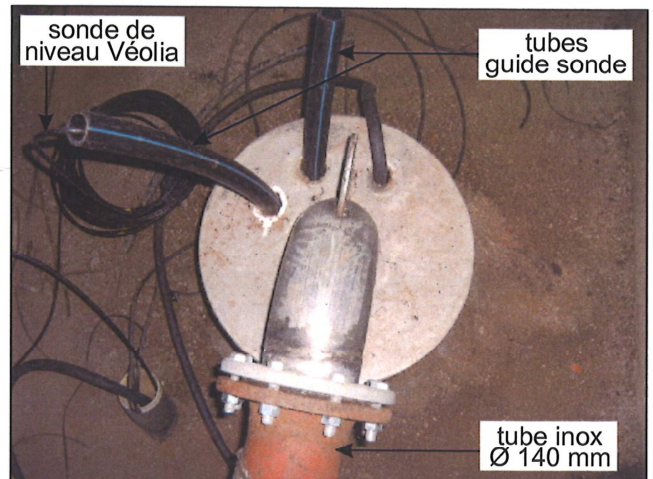
Vues de la tête de forage
