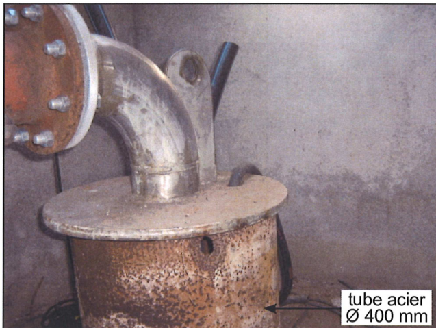
Vues de la tête de forage
