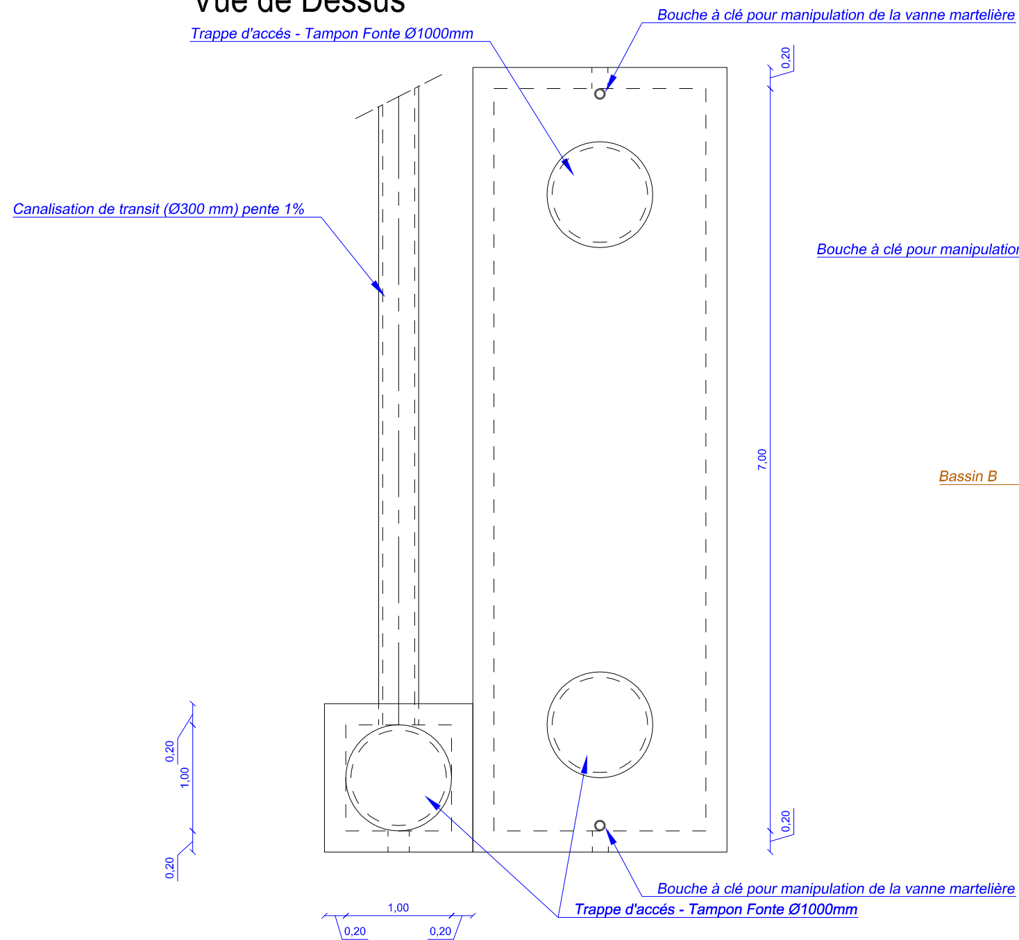
Vue de Dessus
